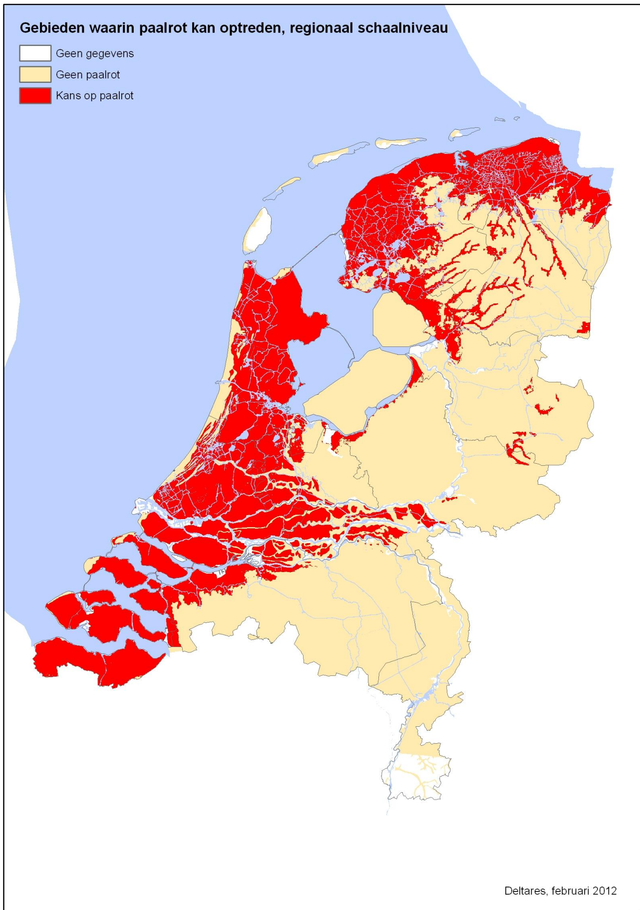
Figuur 4.2 Gebieden waarin paalrot kan optreden.
